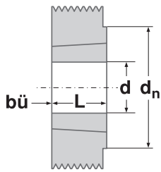
Ausführung Type 1
