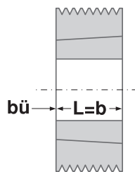
Ausführung Type 5
