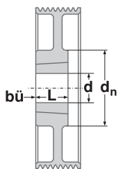
Ausführung Type 4
