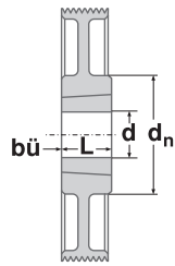
Ausführung Type 2
