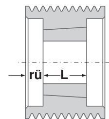
Ausführung Type 6
