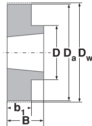
Ausführung Type 8
