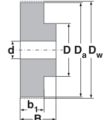
Ausführung Type 6
