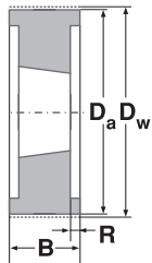
Ausführung Type 4
